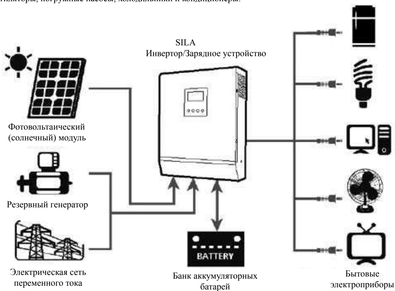
Рис. 1 Схема системы электропитания
